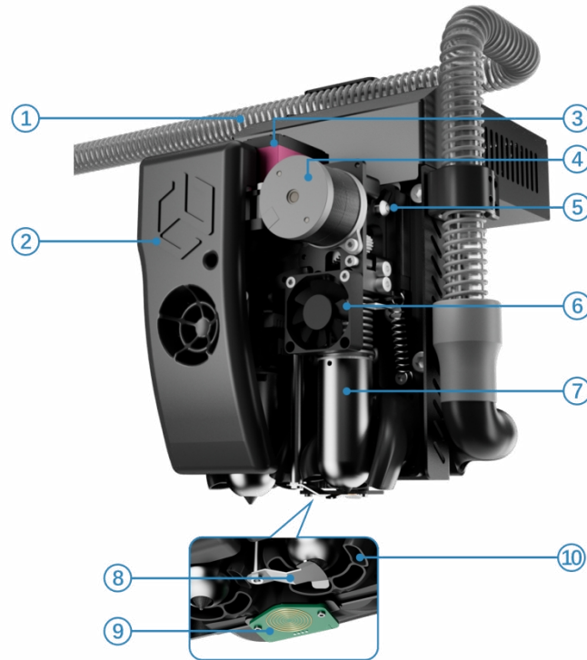
Extruder
